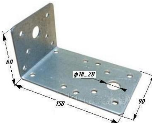
Рисунок А.4 — Внешний вид кронштейна
