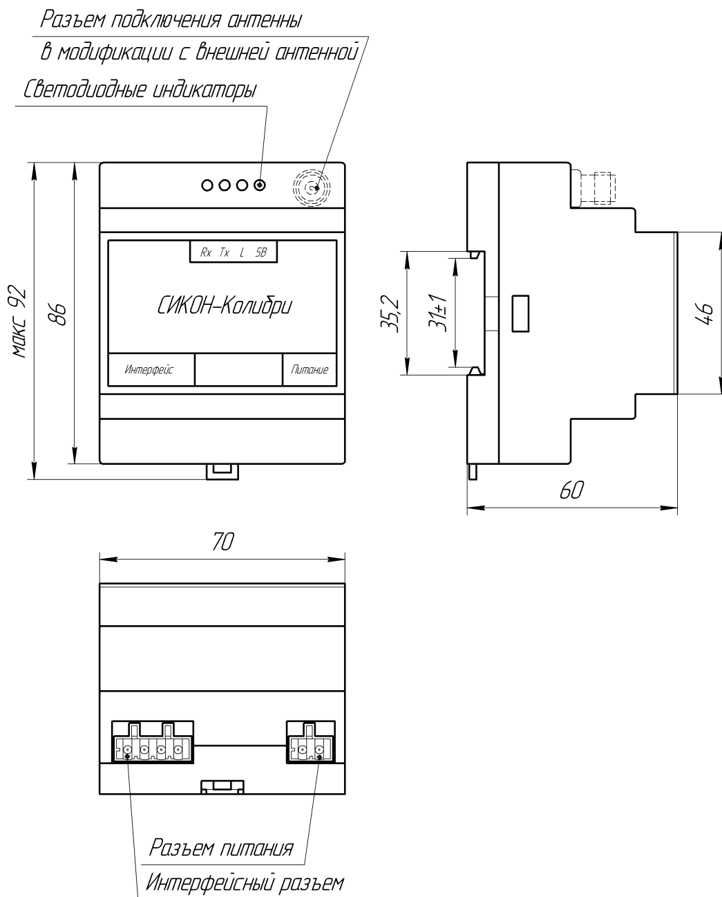
Рисунок А.1 – Внешний вид СИКОН-Колибри.
