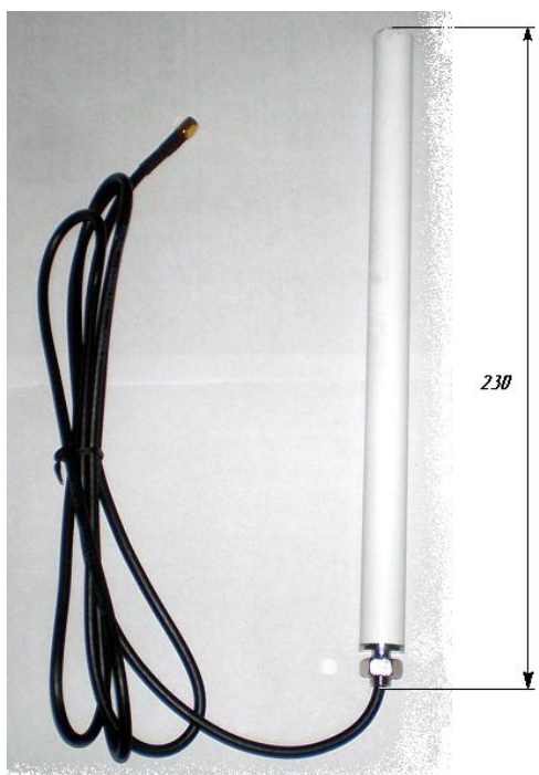
Рисунок А.3 – Внешний вид антенны НМ-Н-001.
