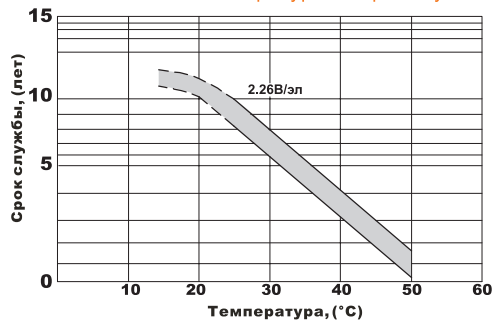
Влияние температуры на срок службы
