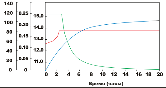
Заряд постоянным напряжением (0.3СА, 25°C)
