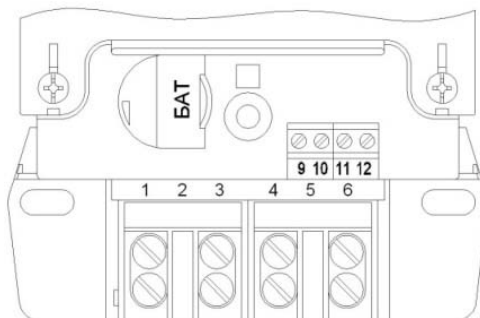
Рисунок 2.1 – Зажимная плата
