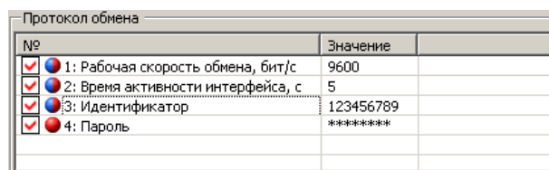
Рисунок 5.17 – Группа параметров «Протокол обмена»
