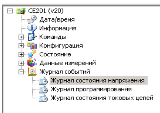
Рисунок 5.32 – Журналы счетчика
