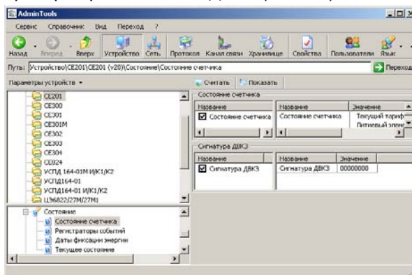
Рисунок 5.30 – Обнуление сигнатуры после срабатывания ДВКЗ
