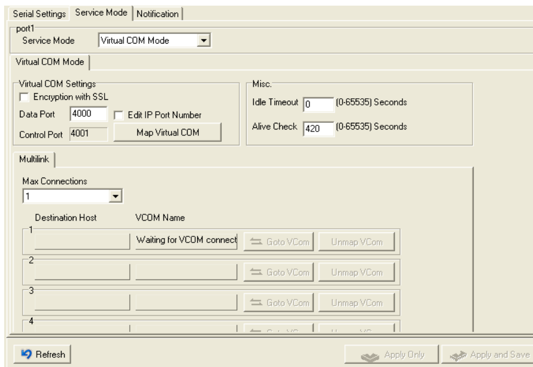
Рис. Virtual COM
