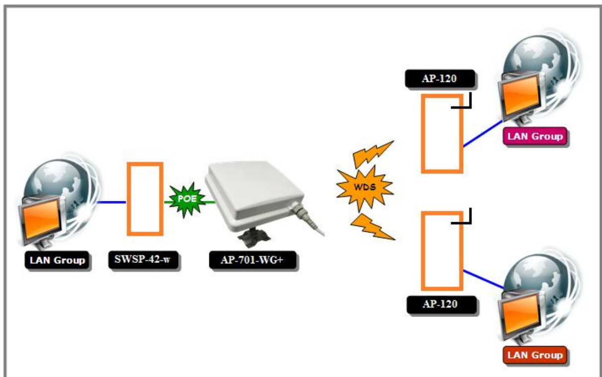
Рис. Режим соединения WDS “точка-многоточка”
