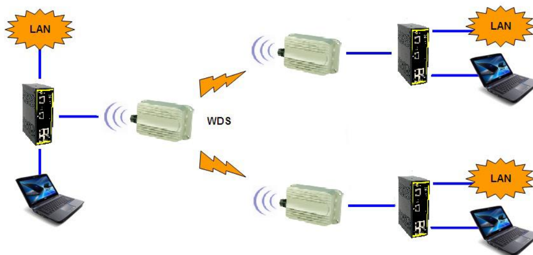
Рис. Режим соединения WDS “точка-многоточка”
